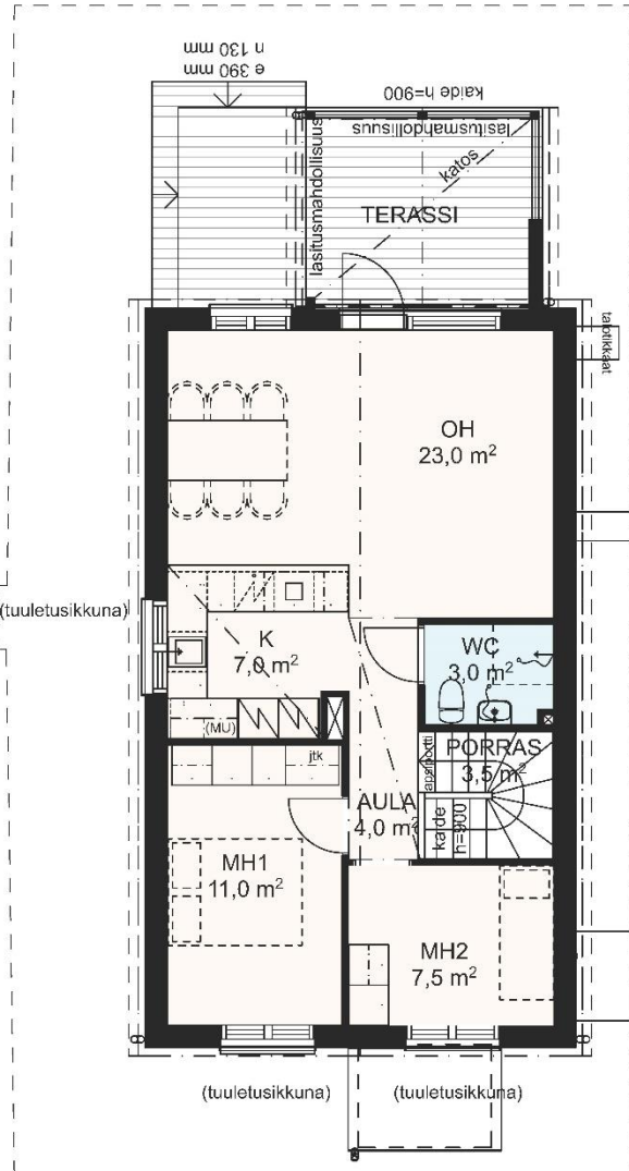
1. kerros
