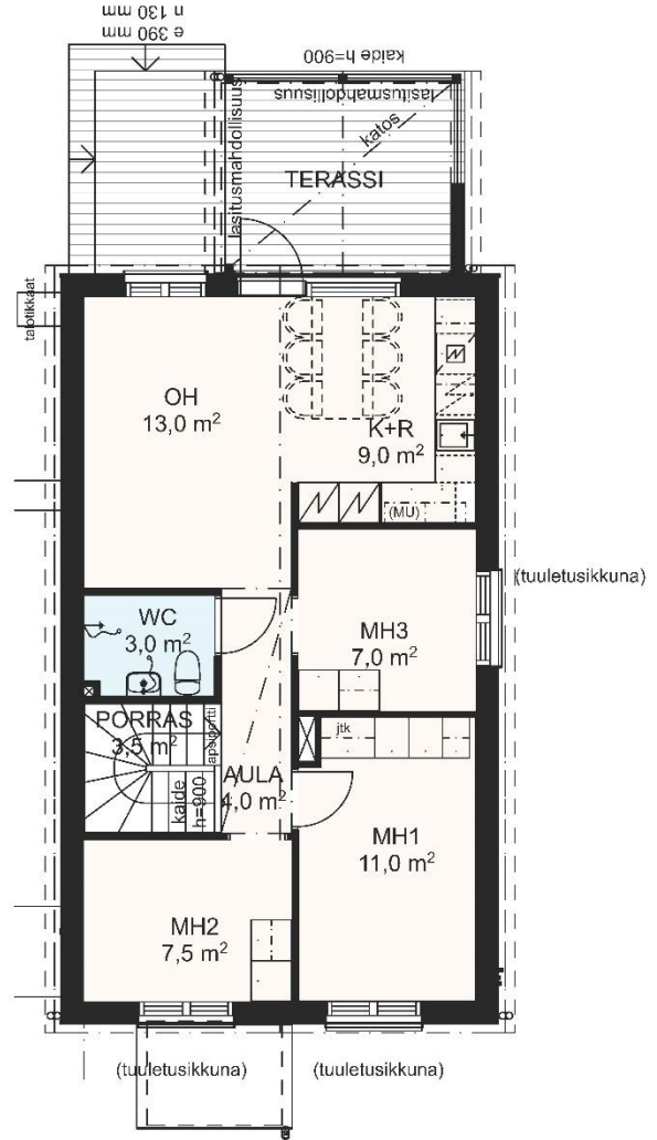
1. kerros
