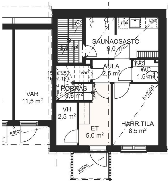
Kellarikerros
