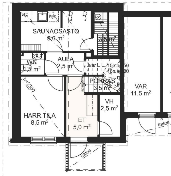
Kellarikerros
